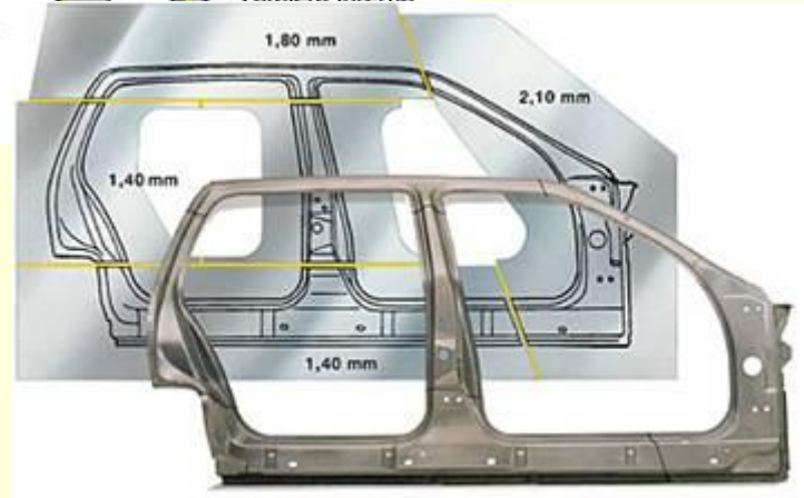
Laterais em 4 espessuras diferentes, soldadas com laser
