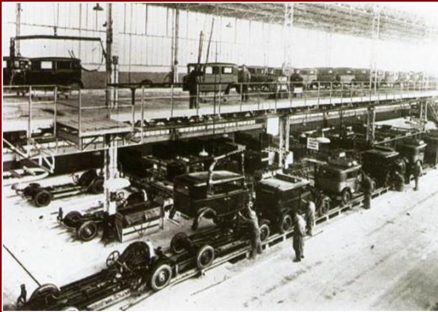
LINHA DE MONTAGEM DE CARROS (segundo F. W. Taylor) FÁBRICAS FORD, EUA, 1915
